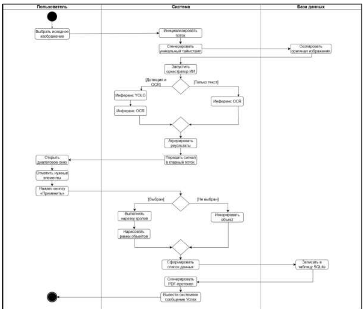
Рисунок 10 – Диаграмма деятельности запустить анализ
