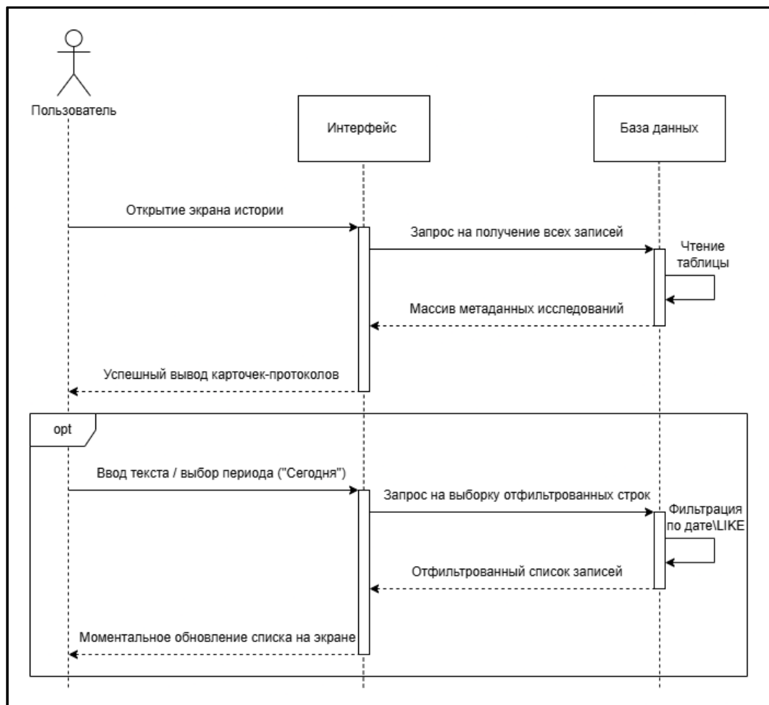
Рисунок 11 – Диаграмма последовательности прецедента посмотреть историю исследований
