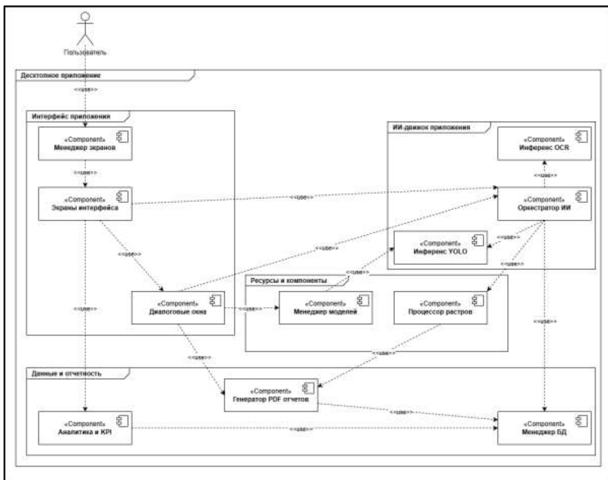
Рисунок 9 – Диаграмма компонентов системы
